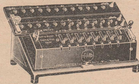
Abb. 2: Unitas mit Schieber-Einstellung 8×7×12×12stellig
