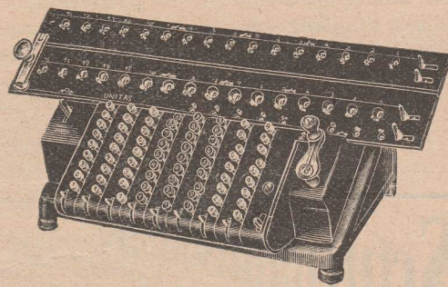
Abb. 4: Unitas mit Tasten-Einstellung 8×9×16×16stellig
