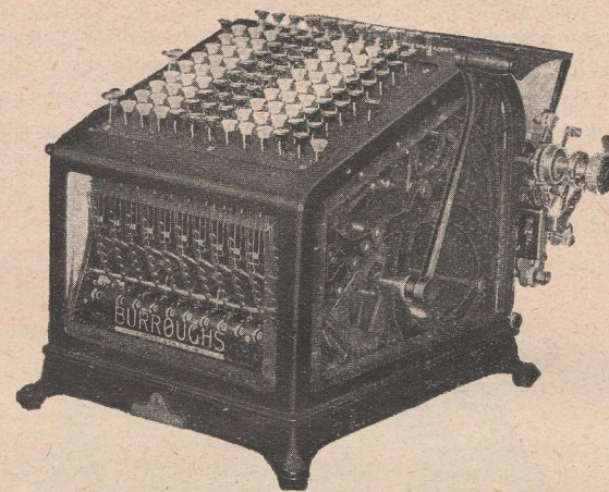
Abb. 1: Selbstschreibende Additionsmaschine
