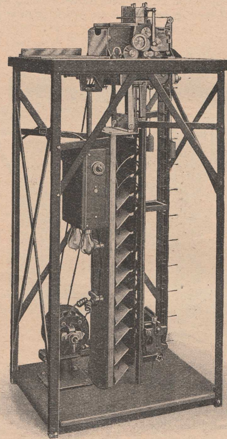
Abb. 3: Sortiermaschine
