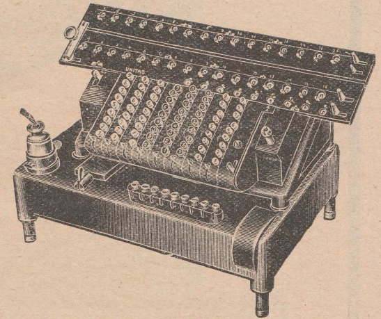
Abb. 6: El. Unitas mit Tasten-Einstellung 8×9×16×16stellig
